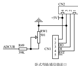
卧式弯插/通信烧录口
