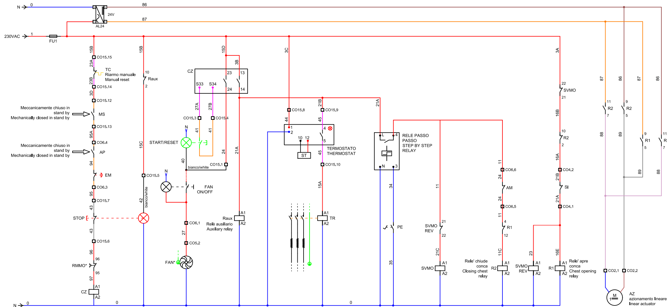
CONFIGURAZIONE INVERTER INVERTER CONFIGURATION
