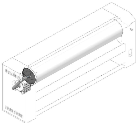
IMPIANTO ASPIRAZIONE SUCTION SYSTEM
