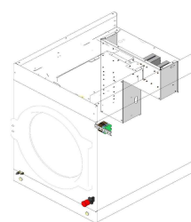
ELETTRONICA ELECTRONICS
