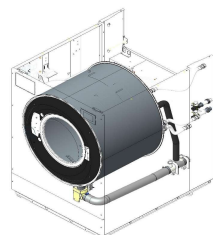
IMPIANTO IDRICO HYDRAULIC SYSTEM
