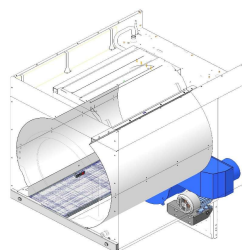
IMPIANTO ASPIRAZIONE SUCTION SYSTEM
