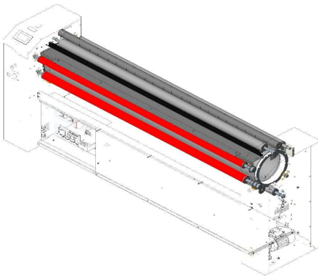
GRUPPO CENTRALE CENTRAL MOVEMENT
