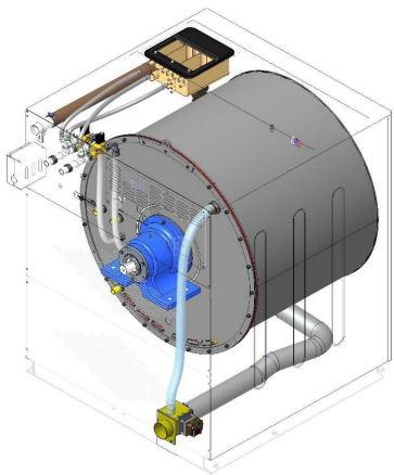
IMPIANTO IDRICO HIDRAULIC SYSTEM
