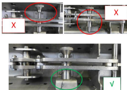
D2W30/55: lato sporco
