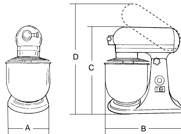
FIG. n°2 - Dibujos del espacio máximo ocupado
