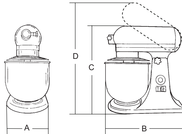
FIG. n°2 - Dimensioni d'ingombro
