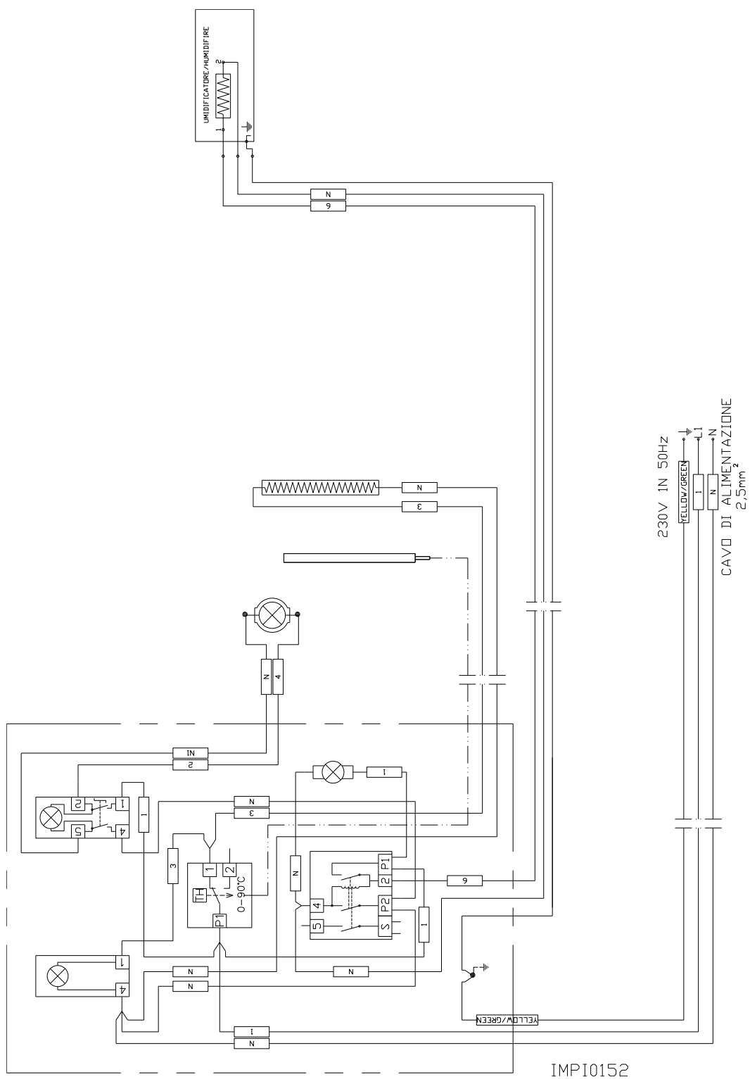
Fig.9.2 Schéma électrique 230 Vac monophasé avec humidificateur (optionnel)
