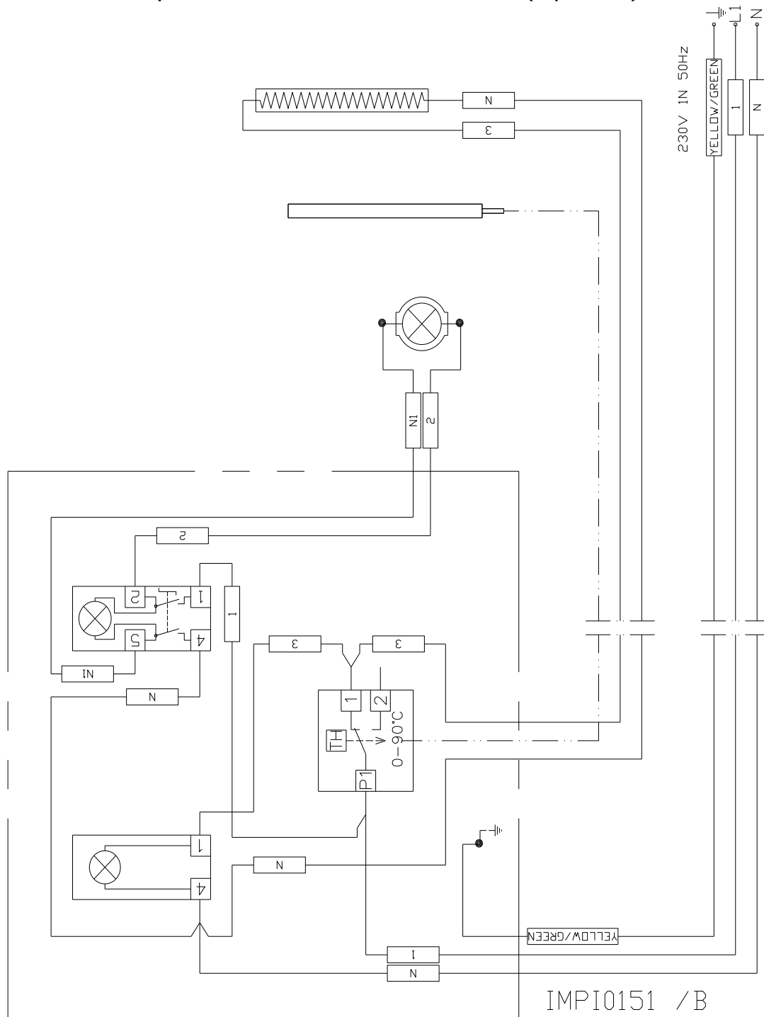
Abb. 9.1 Elektrisches Einphasenschema 230 Vac
