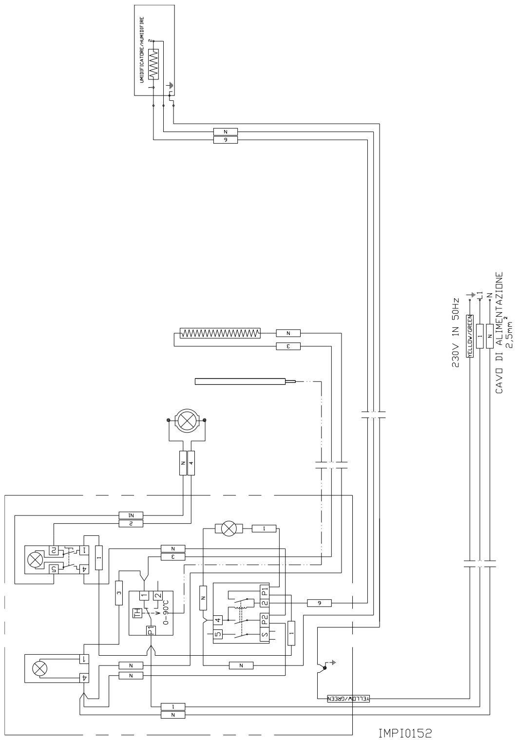
Abb. 9.2 Elektrisches Einphasenschema 230 Vac (Optional)
