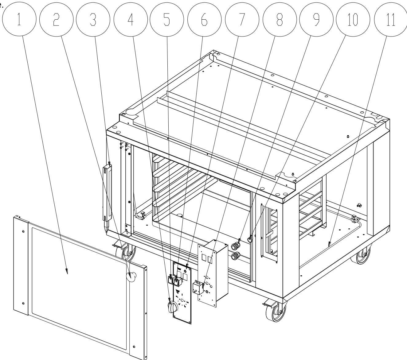
Fig.10.1 Dessin éclaté chambre
