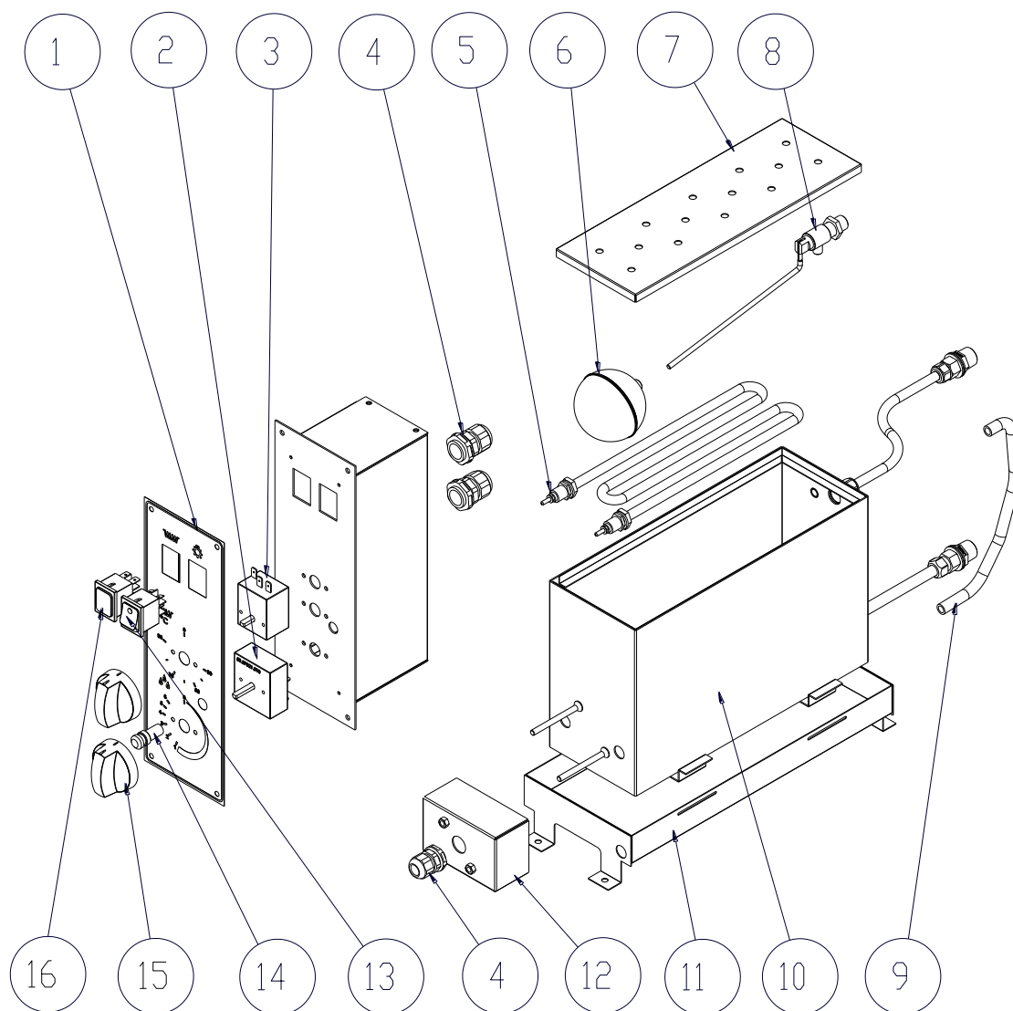
Fig.10.2 Dessin éclaté humidificateur (optionnel)
