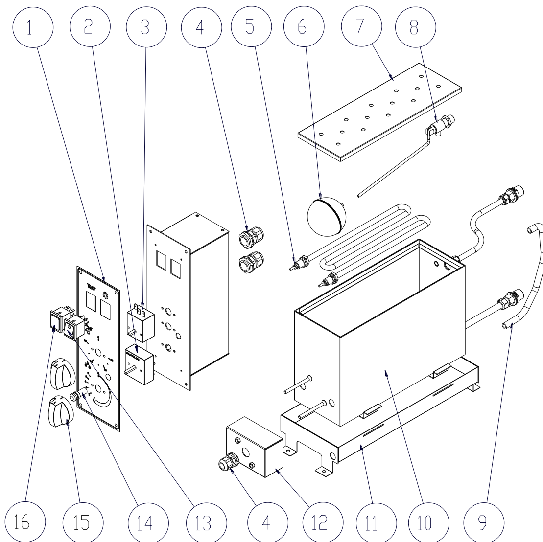
Fig.10.2 Dibujo técnico humidificador (opcional)
