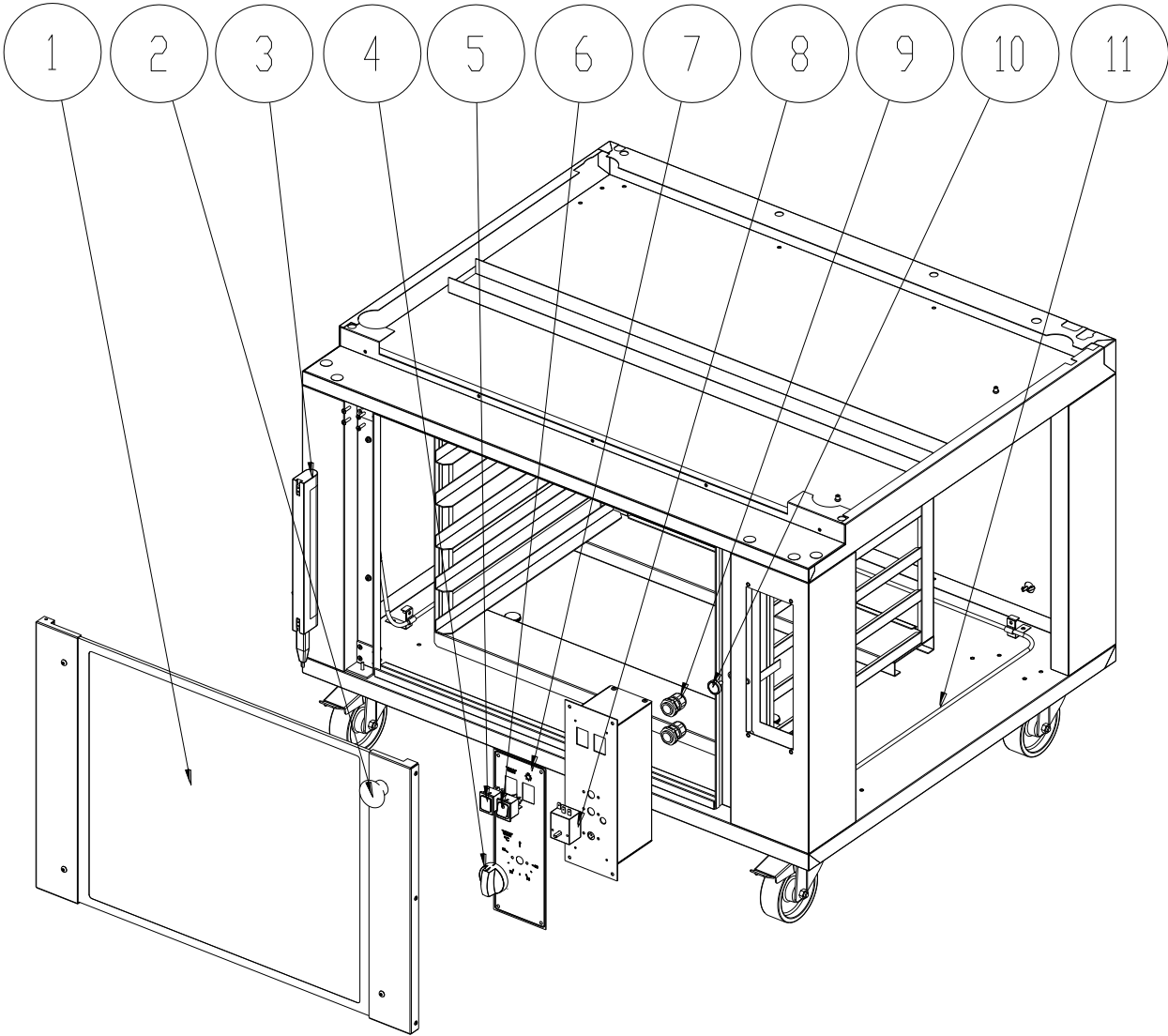
Fig.10.1 Dibujo técnico celda
