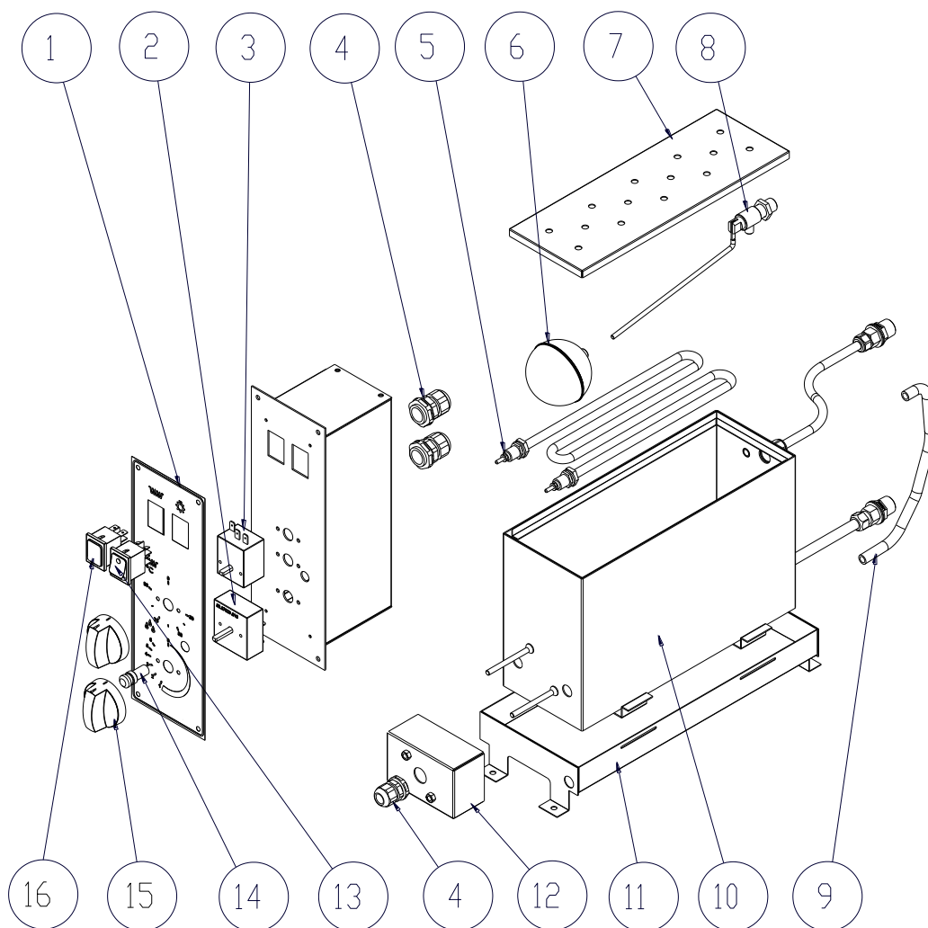
Abb. 10.2 Explosionszeichnungen Bilder des Befeuchters (optional)
