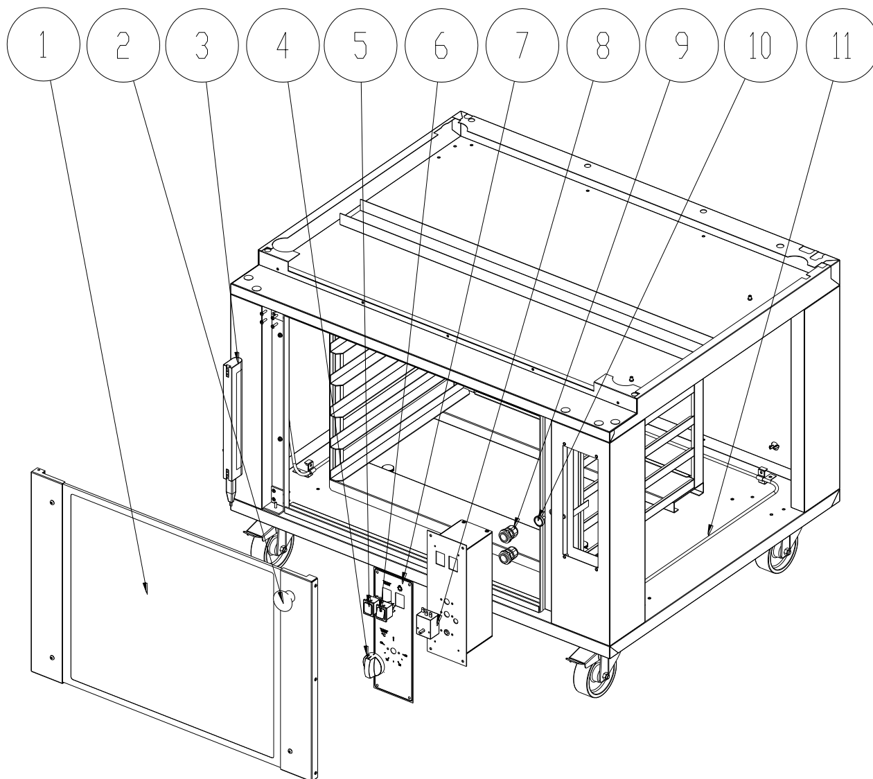
Abb. 10.1 Explosionszeichnungen Bilder
