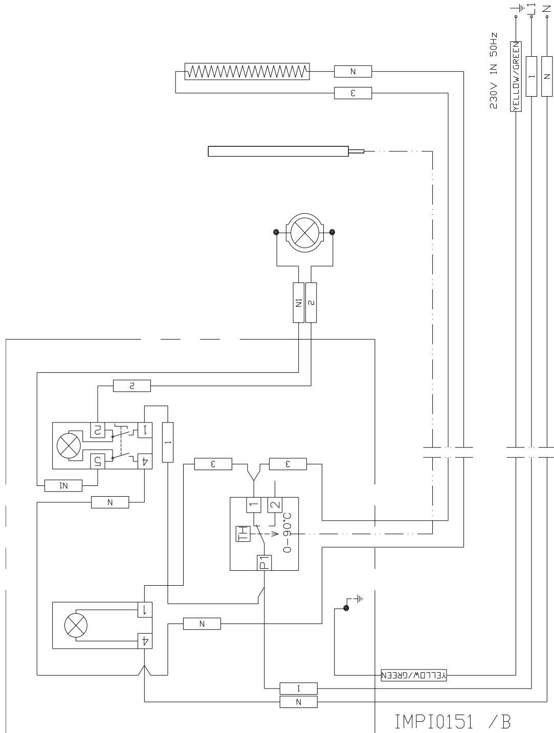
Fig. 9.1 Esquema eléctrico 230 Vac monofásico
