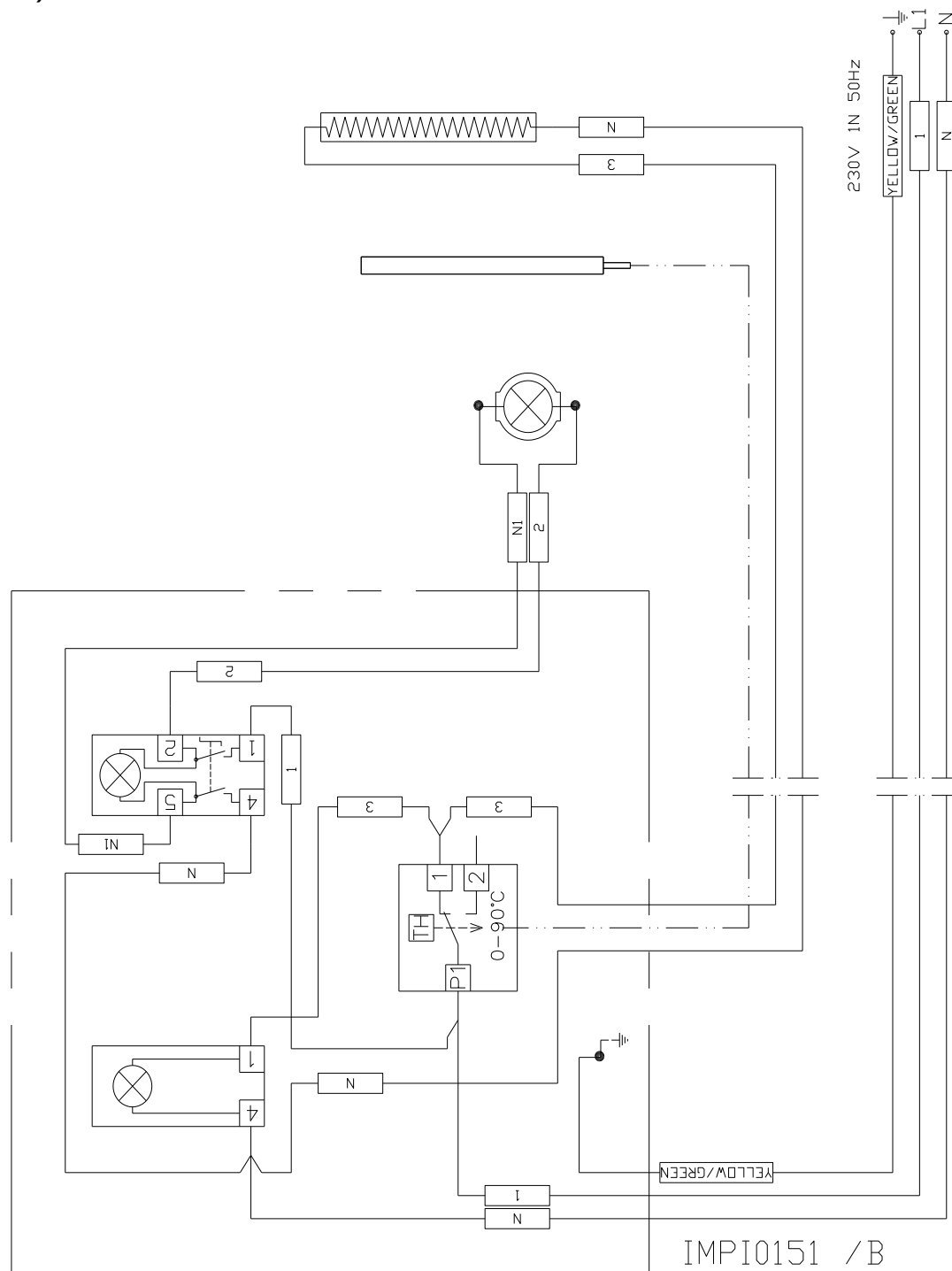
Fig. 9.1 Schema elettrico 230 Vac monofase
