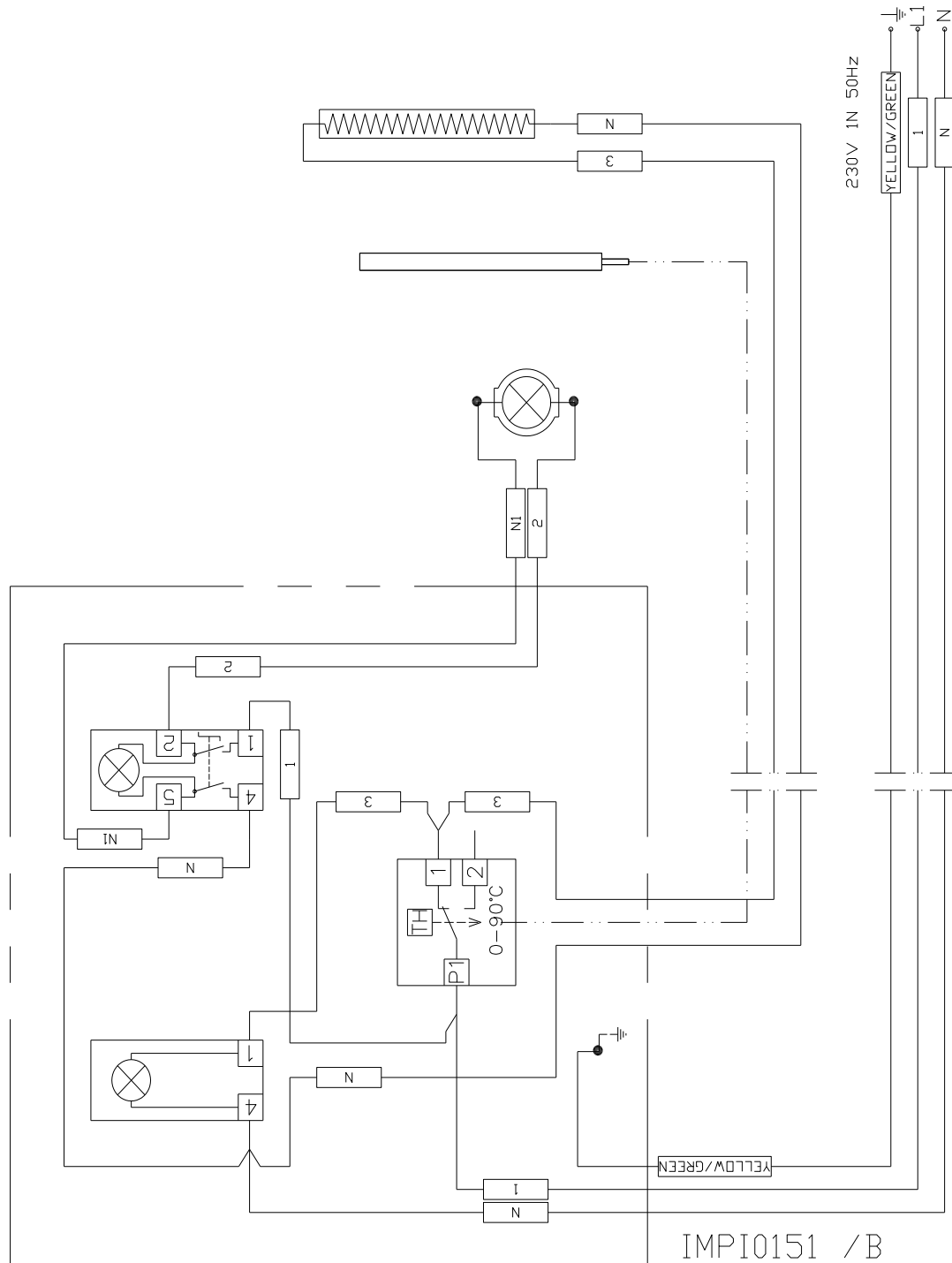
Fig. 9.1 Schéma électrique 230 Vac monophasé
