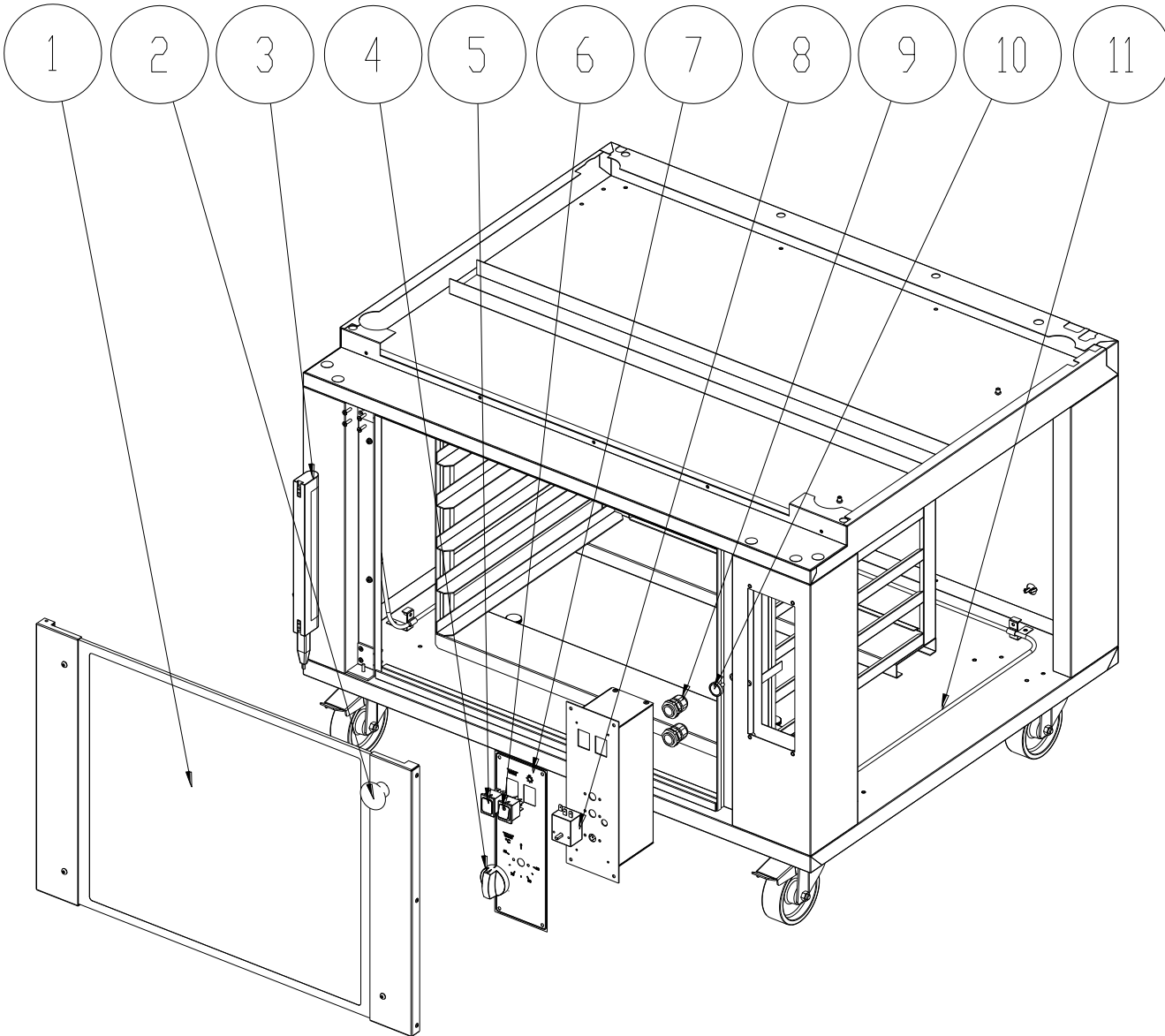
Fig.10.1 Disegno esploso cella
