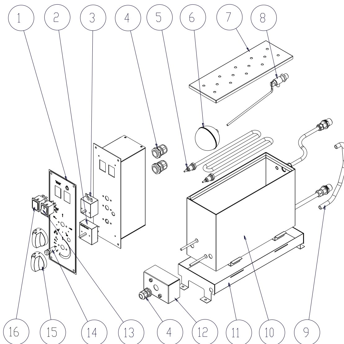
Fig.10.2 Disegno esploso umidificatore (opzionale)
