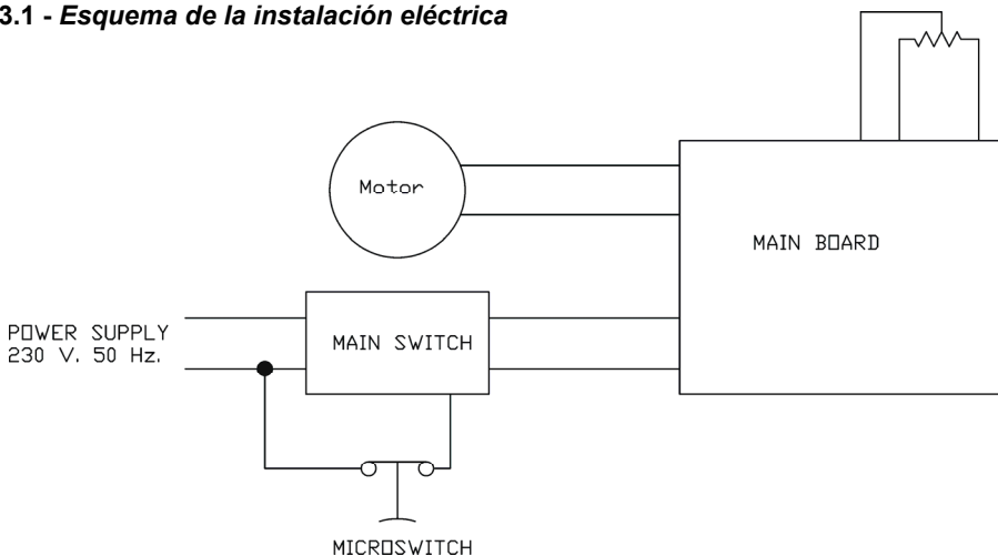
FIG. n°5 - Esquema eléctrico
