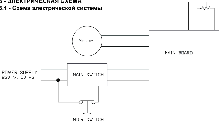
рис. п°5 - Электрическая схема
