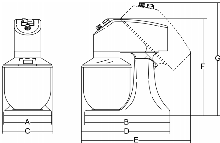
ABB. 2 - Abmessungen über alles
