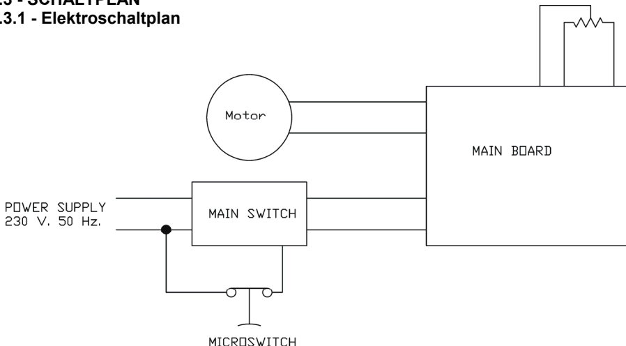
ABB.5 - Elektroschaltplan
