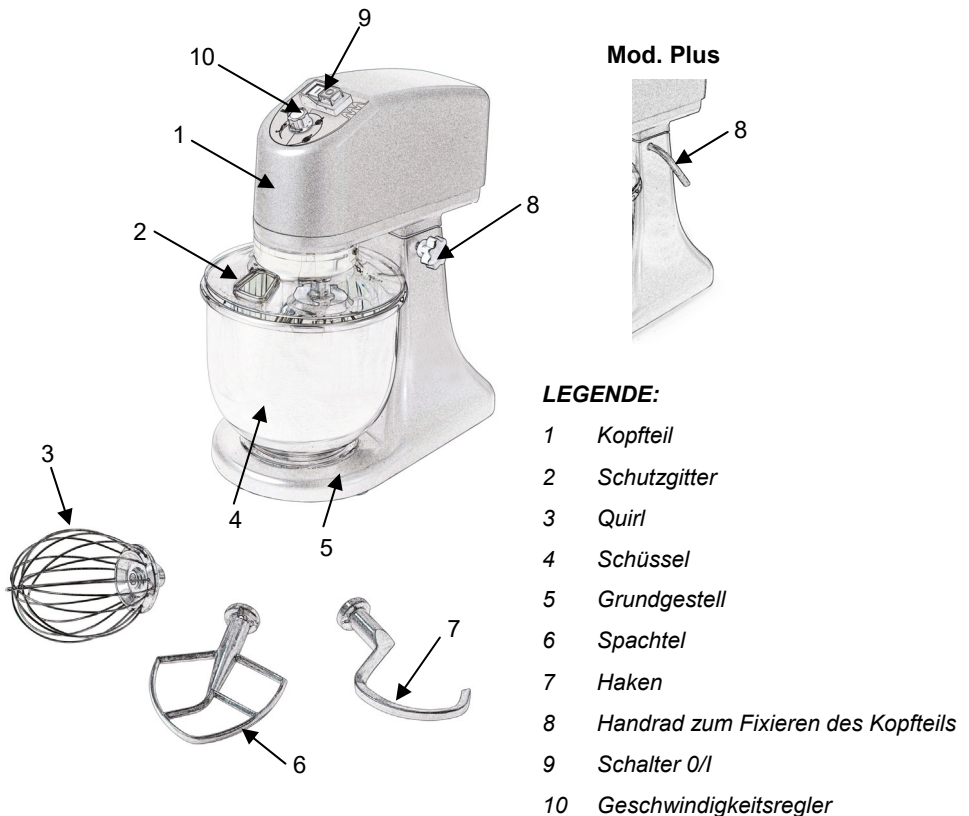
ABB. 1 - Gesamtansicht des Gerätes
