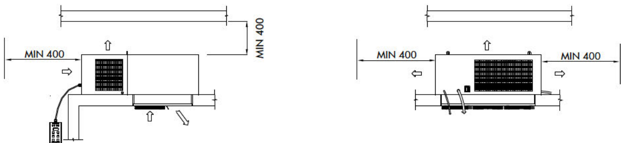
Figure 3 – Cotes minimales à respecter.
