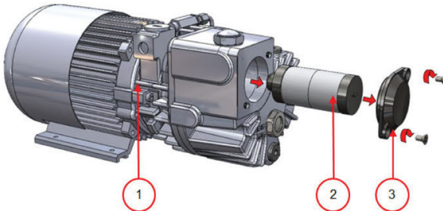
Schéma 12 : Remplacement du filtre à échappement d'air
